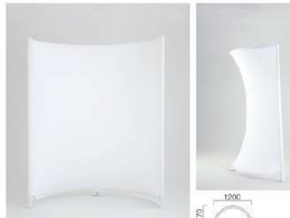
PW-045A スクリーンパーテーション [1200] Screen Partition W1200 D670 H1500 生地:ホワイト、ポリエステル フレーム:ホワイト、スチール
