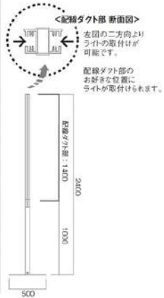
LI-77 配ダクトライトスタンド [1000] Light Stand With Wiring Duct φ500 H2400 ブラック、スチール ・配線ダクト 100V 仕様 ・40W スポット 12 灯まで取付可
