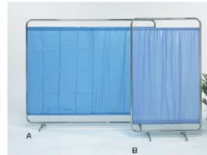
PW-35A・B スクリーン Screen Partition A [3200] B [2800] A:W1800 H1515 B:W900 H1515 カーテン:ブルー、ナイロン 防炎加工 フレーム:グロームメッキ 脚:アルミ
