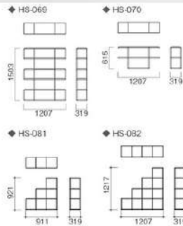
HS-070 ユニットディスプレイ台 Unit Display Stand [10606] W1207 D319 H615 天板ホワイト、デコラ フレームクロームメッキ
