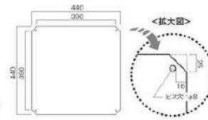
◆ パネル素材は樹脂性。化粧ビスでフレームに固定します。
