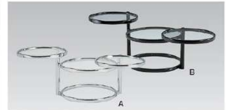
T-194A-B トリプルテーブル [4993] Triple Tier Table W590~1380 D500~845 H435 天板Aクリアガラス (太さ470、小φ375) Bクリアガラス (太さ470、小φ375) 脚部Aクロームメッキ B:ブラック、スチール
