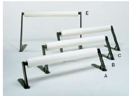
C-422A-B-C-E パイプベンチ [3000] Pipe Bench φ150 W1500 A:D400 H400 B:D500 H500 C:D600 H550 E:D900 H800 座面:ホワイト, レザー フレーム:ブロンズメッキ
