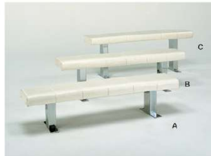
C-424A-B-C スリムベンチ [4000] Slim Bench W1500 D300 A:H340 B:H440 C:H550 座面:ホワイト, レザー フレーム:クロームメッキ
