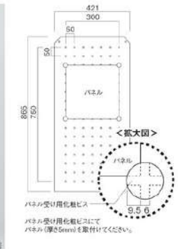
◆拡大図◆ パネル受け化粧ビスにて パネル(厚5mm)を取付けてください。
