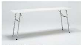
T-235 会議用テーブル [3204] Simple Conference Table W1800 D450 H730 天板ホワイト、デコラ 脚部ステンレス
